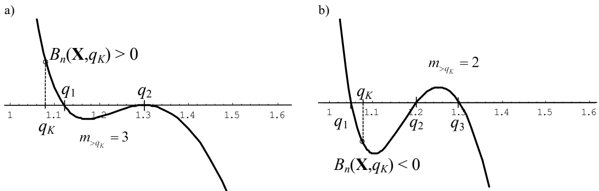
Abb. 2 Der Graph der Barwertfunktion q \mapsto B_n(\mathbf{X}, q) einer a) vorteilhaften Investition X mit ungerader rechtsseitiger Gesamtvielfachheit m_{>q_K} und b) unvorteilhaften Investition X mit gerader rechtsseitiger Gesamtvielfachheit m_{>q_K}
